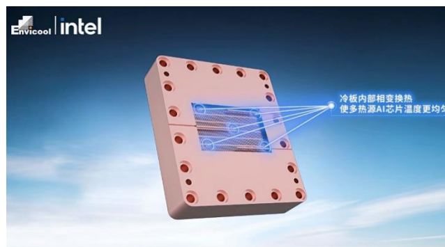
图表 9：两相冷板液冷方案
