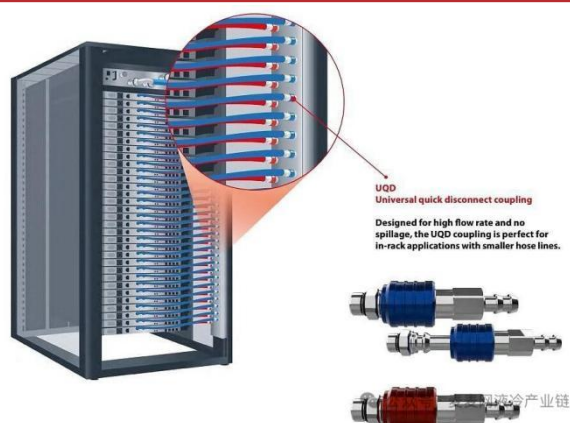
图表 4: UQD 安装位置
