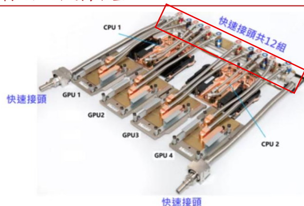
图表 5: NVQD 安装位置
