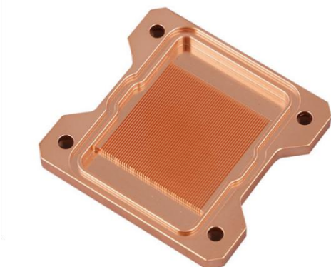
图表 2：冷板铲齿结构
