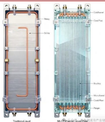
图表 8：微通道液冷板
